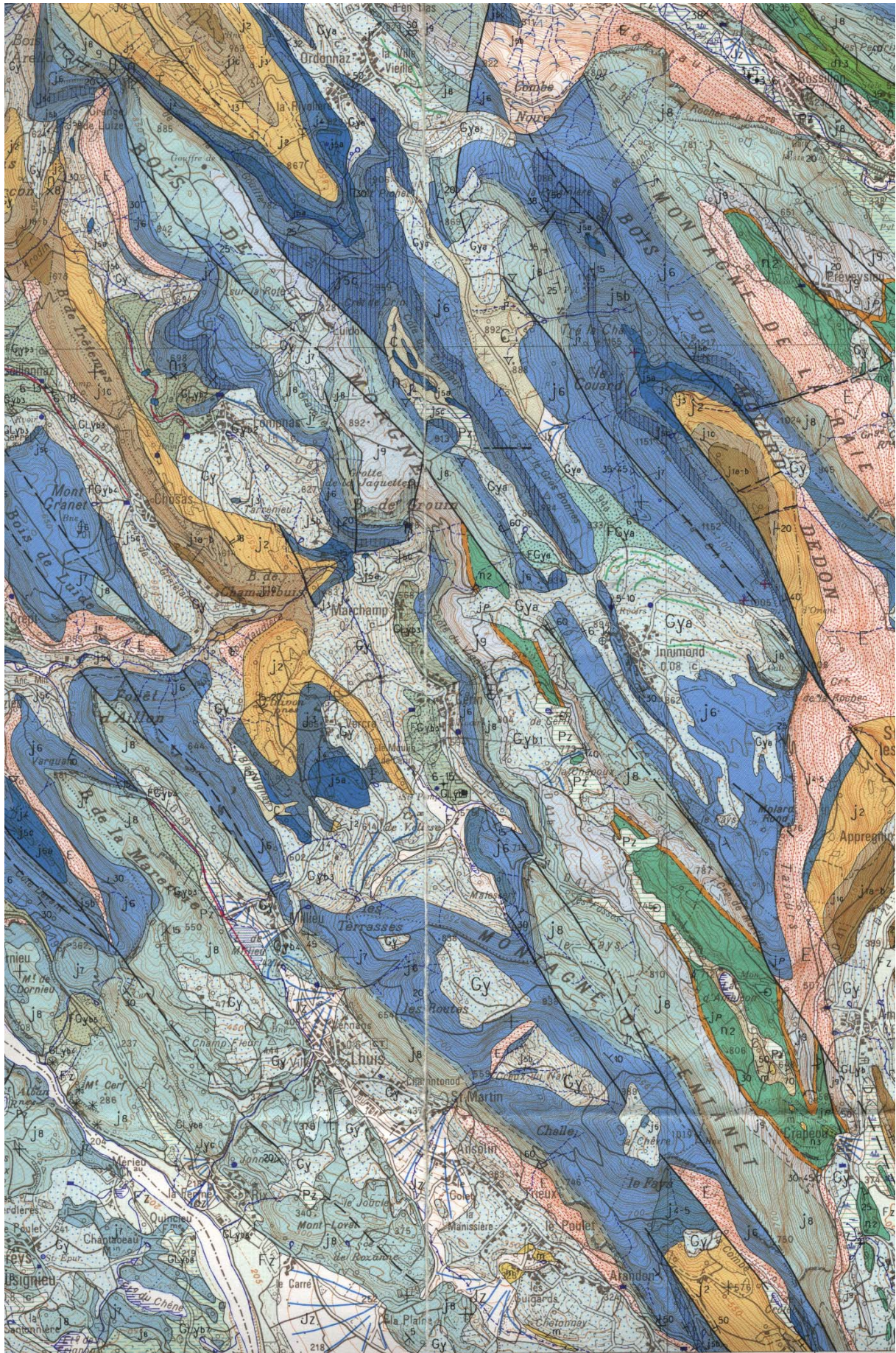
Extrait carte géologique Belley – 1/50000
