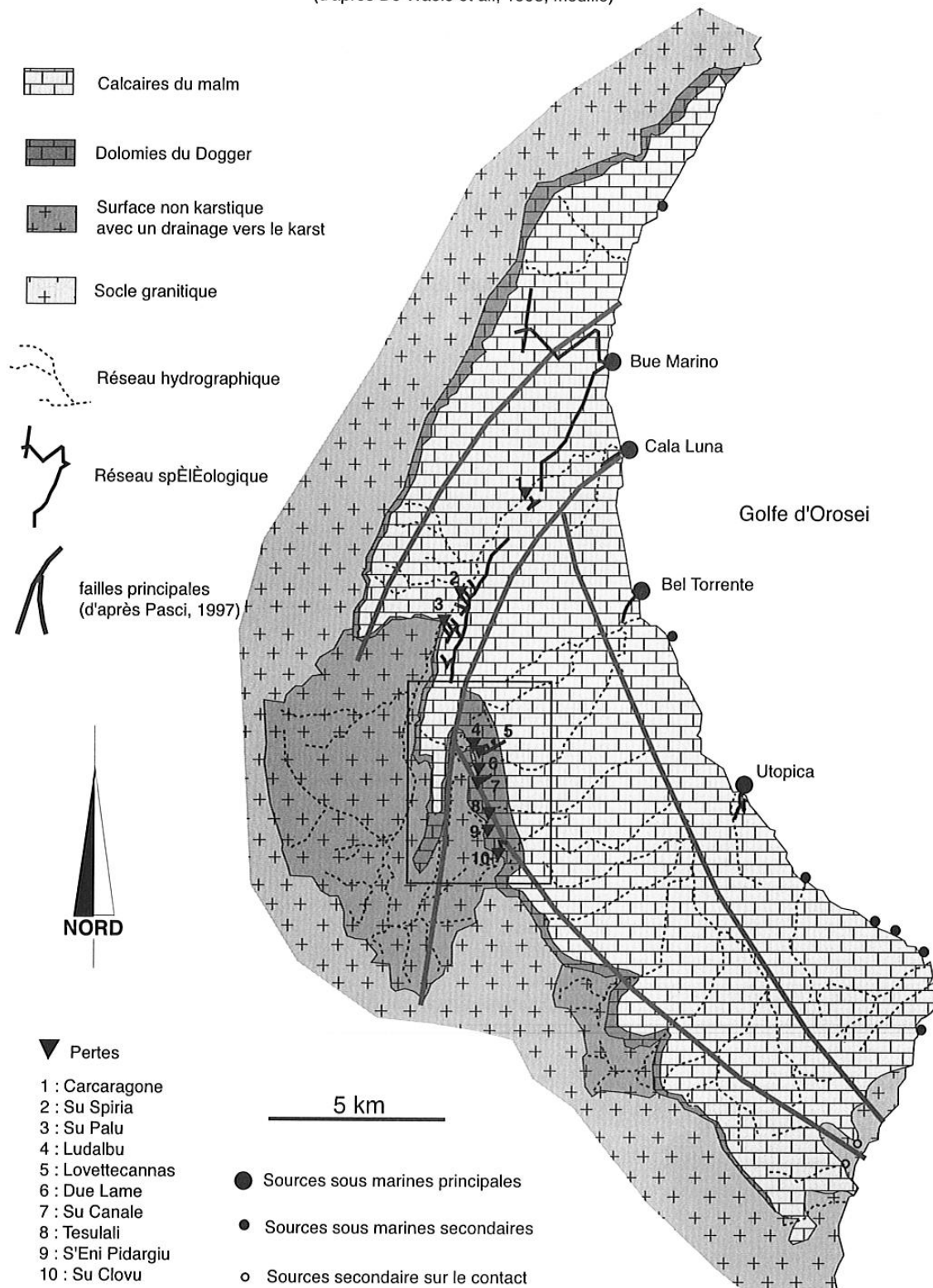
FIG.2 : CARTE GEOLOGIQUE ET HYDROGEOLOGIQUE SIMPLIFIEE DU SUPRAMONTE DE BAUNEI : LOCALISATION DE LA ZONE DE RECHERCHE (d'après De Waele et al., 1995, modifié)
